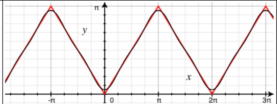
Ici on a tracé f et la série de Fourier jusqu'à l'harmonique de rang 3
