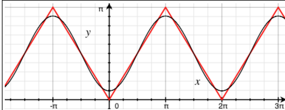
Ici, on a tracé f et le fondamental.
