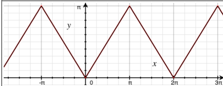
Enfin, ici on a tracé f et la série de Fourier de f jusqu'à l'harmonique de rang
